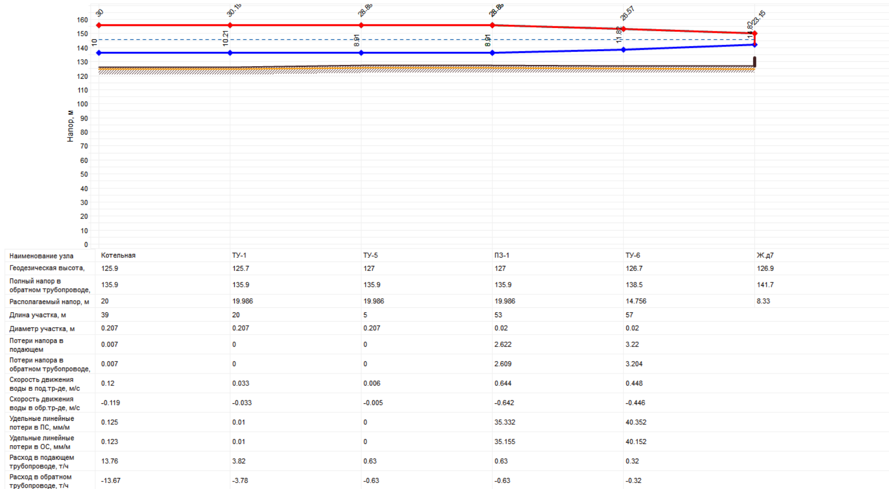
Рисунок 1.2- Результаты гидравлического расчета, пьезометрический график от котельной «ПУ-1» (новое строительство)
