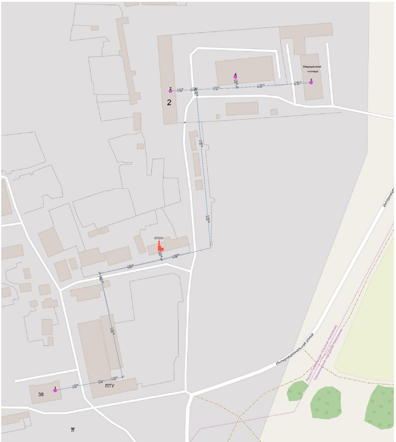
Схема 1.1- Общий вид рабочего экрана электронной модели системы теплоснабжения котельной ПУ-1 (новое строительство)
