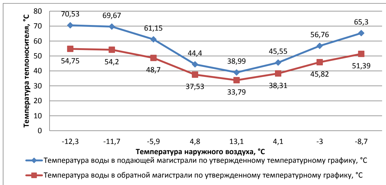
Рисунок 1.3. – Среднемесячные температуры наружного воздуха и теплоносителя.
